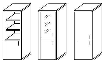
A.СУ-1.1 Л/Пр A.СУ-1.2 Л/Пр A.СУ-1.3 Л/Пр размеры 403x365x1975
