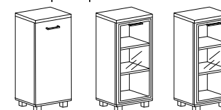
KSU-2.3 KSU-2.4 KSU-2.4R размеры 400x430x1260
