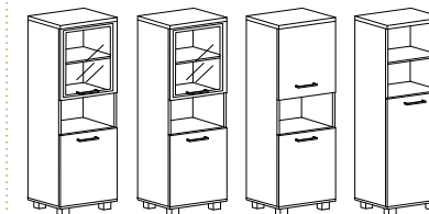
KSU-1.1 KSU-1.2 KSU-1.2R KSU-1.3 размеры 400x430x2060
