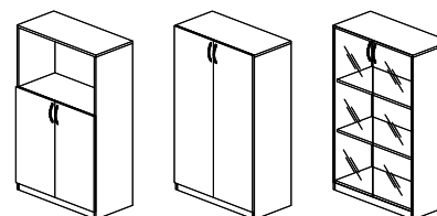
В.СТ-2.1 В.СТ-2.3 В.СТ-2.4 770x359x1203
