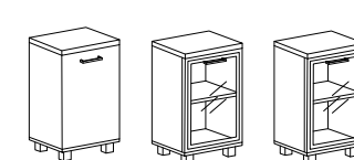
KSU-3.1 KSU-3.2 KSU-3.2R размеры 400x430x960
