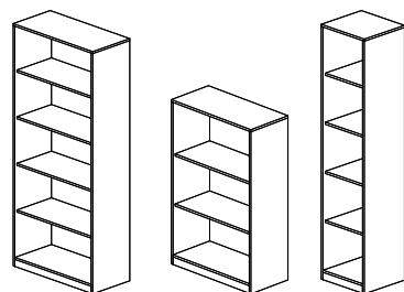
В.СТ-1 770x359x1914 В.СТ-2 770x359x1203 В.СУ-1 388x359x1914
